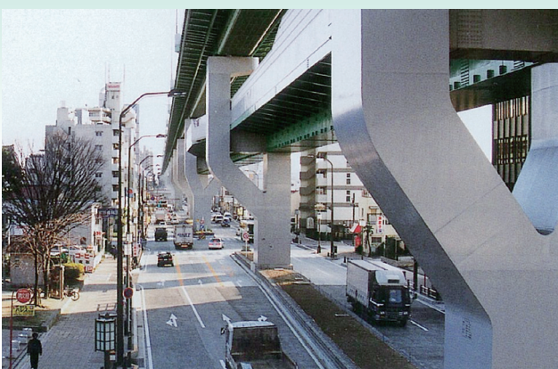
高速 1 号楠線 Y 型 2 層構造
