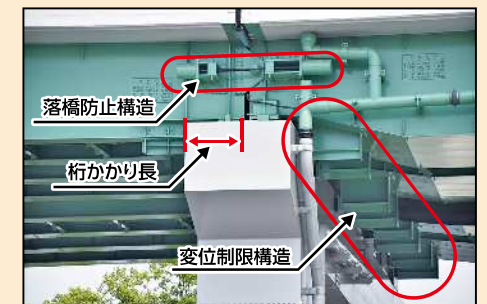
③橋桁の落橋防止システム
