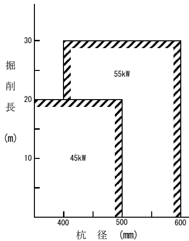
図2.1 アースオーガの選定
