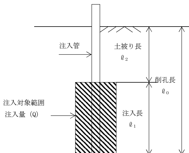
図8.2 施工図
