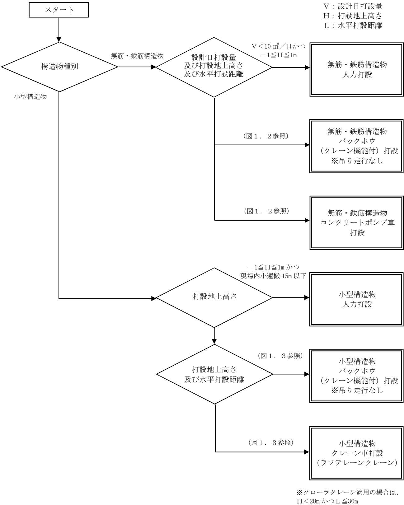
図1.1 コンクリート打設工法の選定
