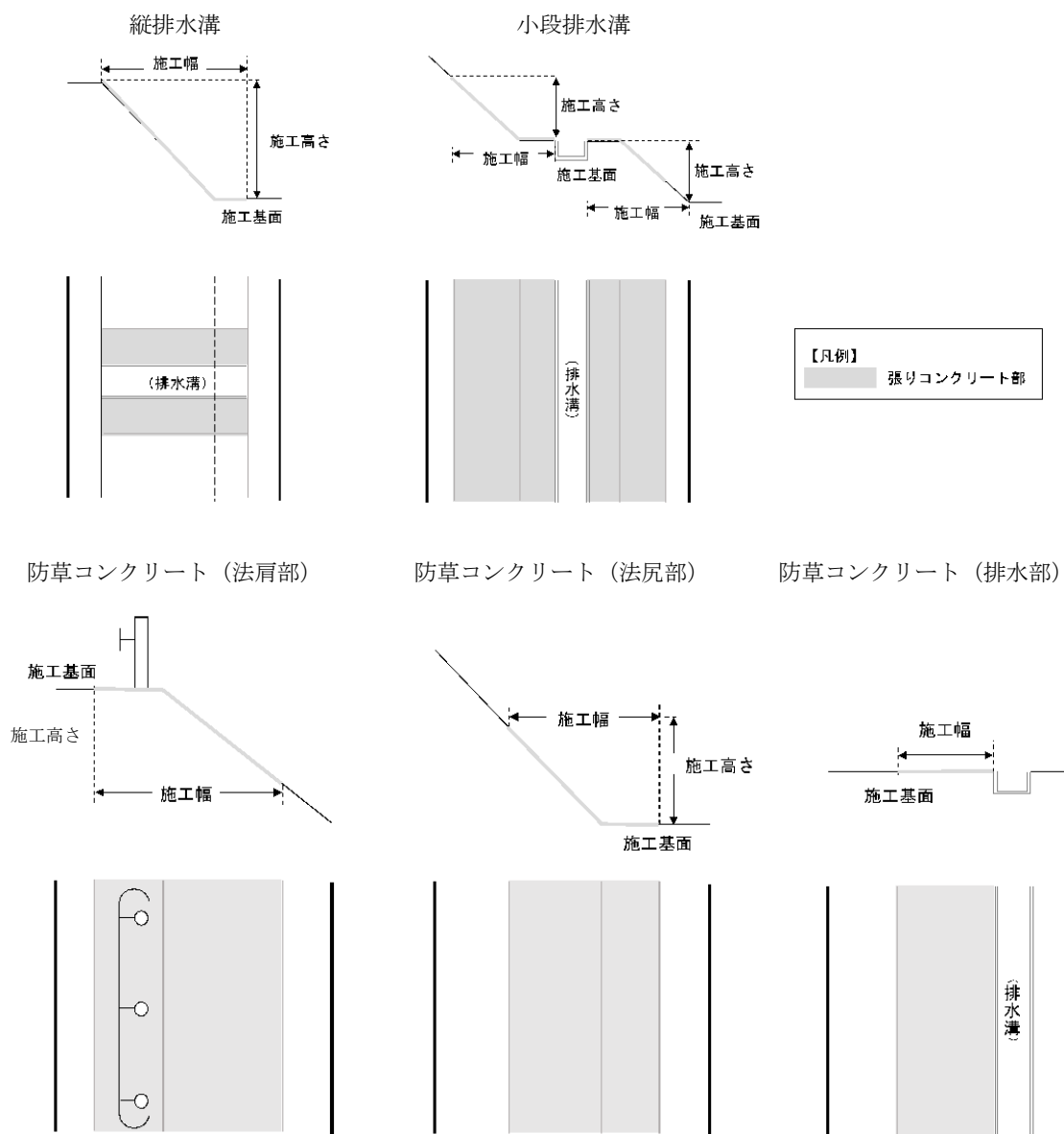
図4. 1 張りコンクリートの例
