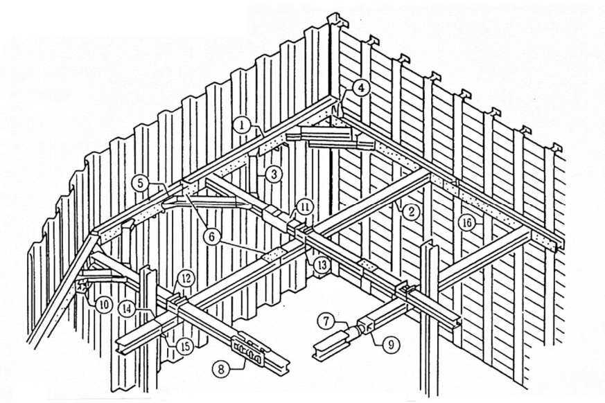
図8.1 土留標準図
