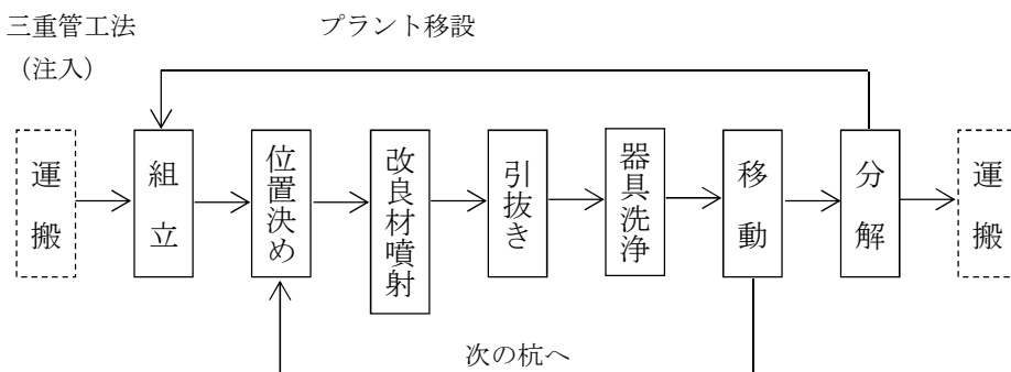
図8.1 施工フロー図
