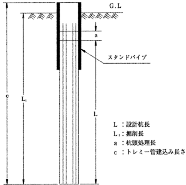
図1.1 施工図
