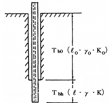
図3.2 施工状況 (プレボーリング)
