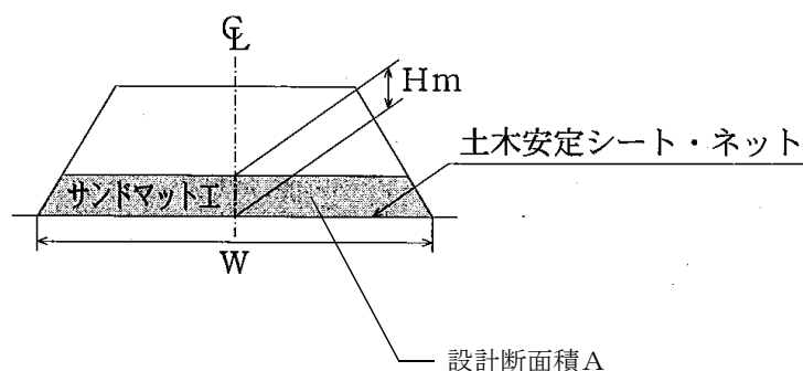
図 6. 1 施工図
