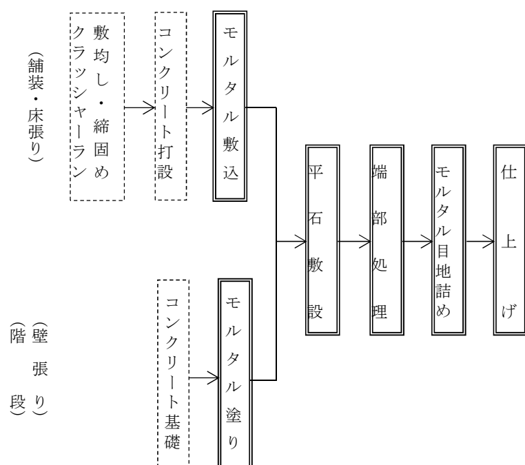
図3.1 施工フロー
