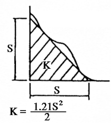
すみ肉溶接図
