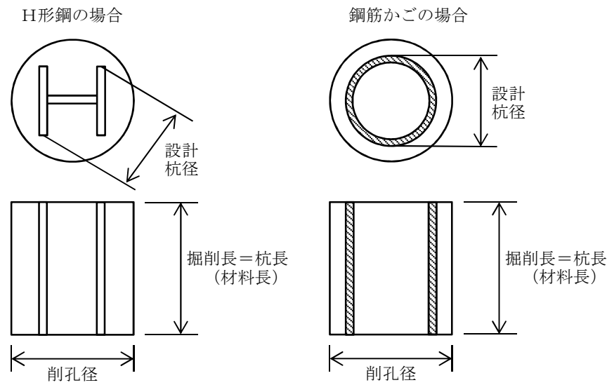
施 工 図
