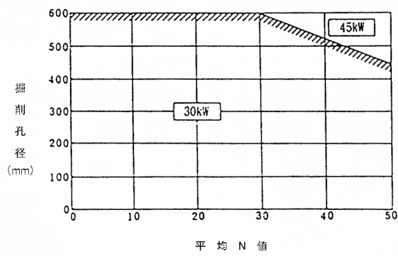
図3.1 アースオーガ規格選定図
