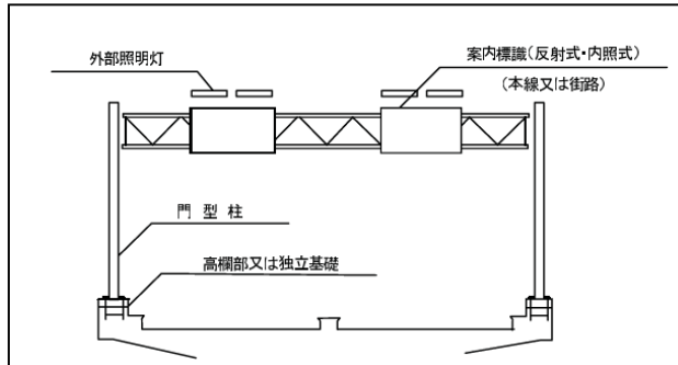
(1) 門型 (案内標識)
