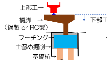
杭基礎・フーチング形式
